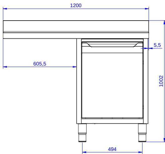
Sivulta
